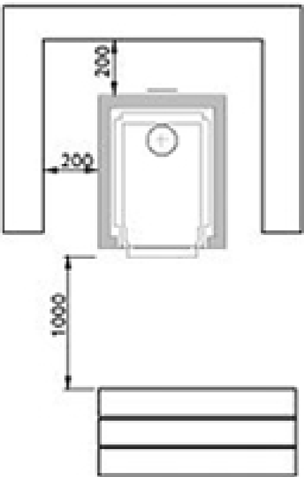
palava rakenne/brännbart material Конструкции из горючих материалов
